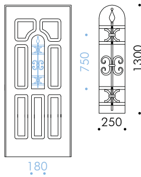
Grata 900-C 25x130 rA
