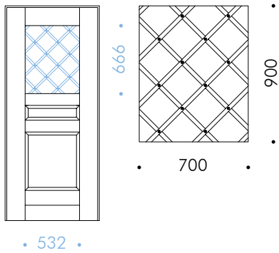
Grata CHIODATA "D" 70x90
