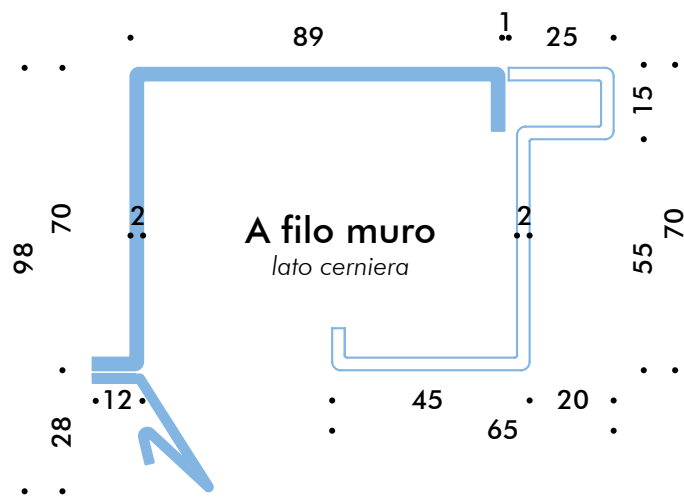
A filo muro
