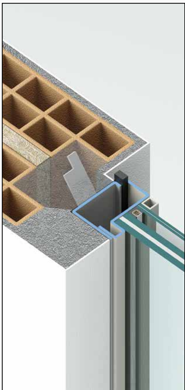
Cassamatta : B1, rifinitura muro ad intonaco.
