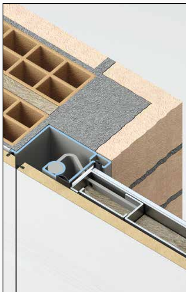
Cassamatta : A Boiserie, rifinitura muro esterna con mattoni a faccia vista.
