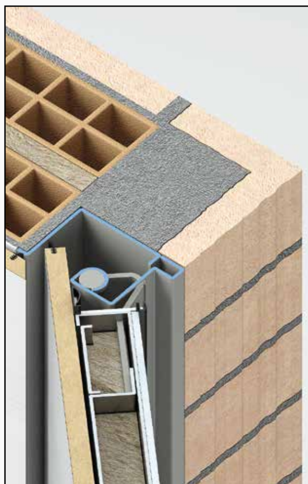
Particolare : porta blindata in apertura.
