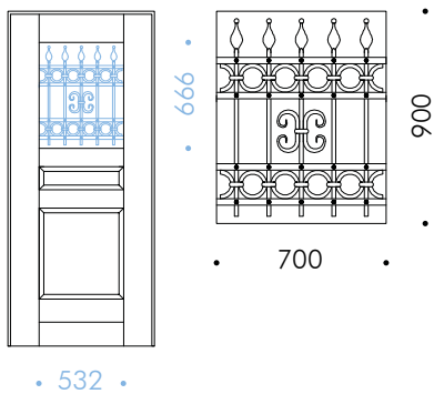
Grata 900-C 70x90
