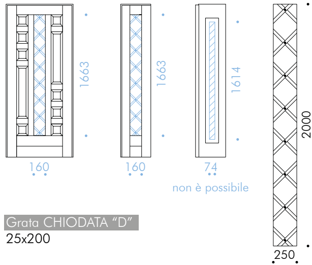
Grata CHIODATA 25x200
