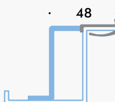
48 60 telaio maggiorato
