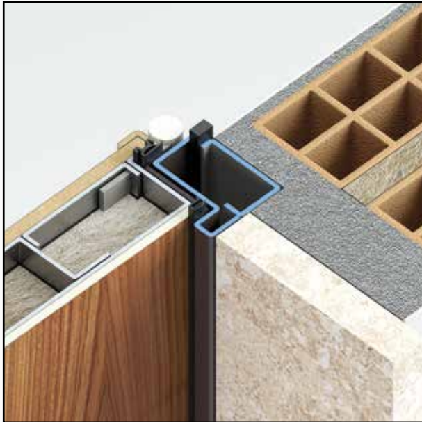
Cassamatta : B, rifinitura esterna con stipiti in marmo.
