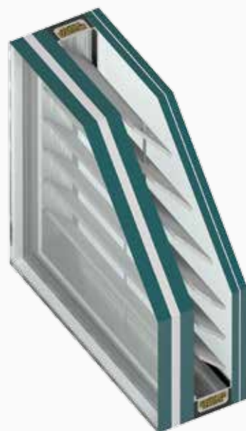
Sezione vetrocamera P50 + veneziana
