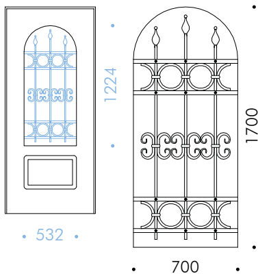
Grata 900-C 70x170 rA
