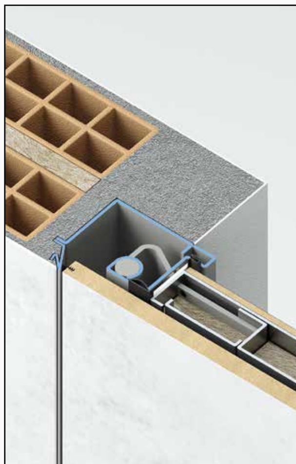
Cassamatta : A Filo muro, rifinitura muro ad intonaco.
