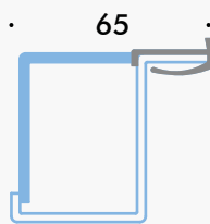
65 45 telaio standard
