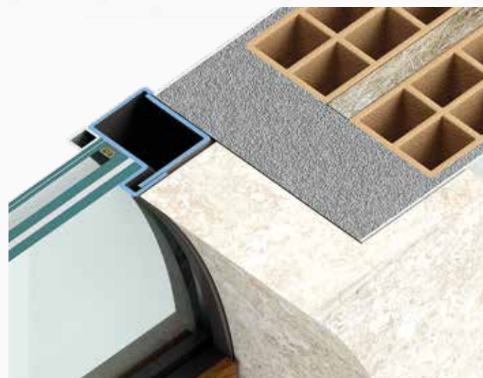
SEZ. 2 : lucernario ad arco vetrocamera P20.
