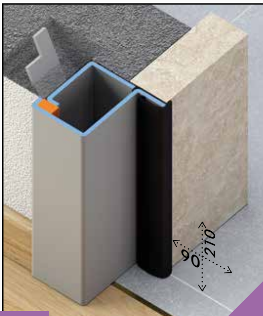
POSA FILO INTERNO
