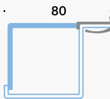
80 60 telaio compensativo
