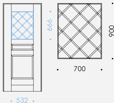
Grata FORATA "D" 70x90
