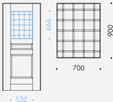
Grata FORATA 70x90
