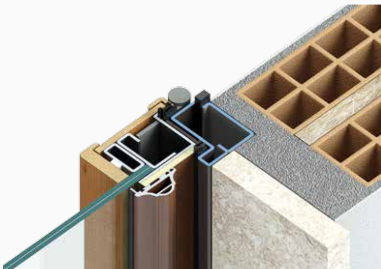
SEZ. 2 : anta piccola, muro, antisfondamento 10/11.
