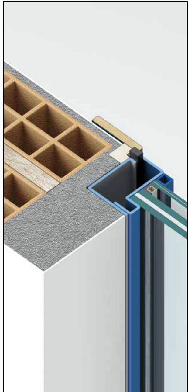
Cassamatta : BIM, rifinitura muro ad intonaco con mostra interna che copre in parte il telaio.
