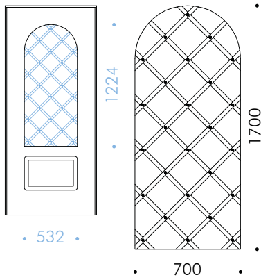
Grata CHIODATA "D" 70x170 rA
