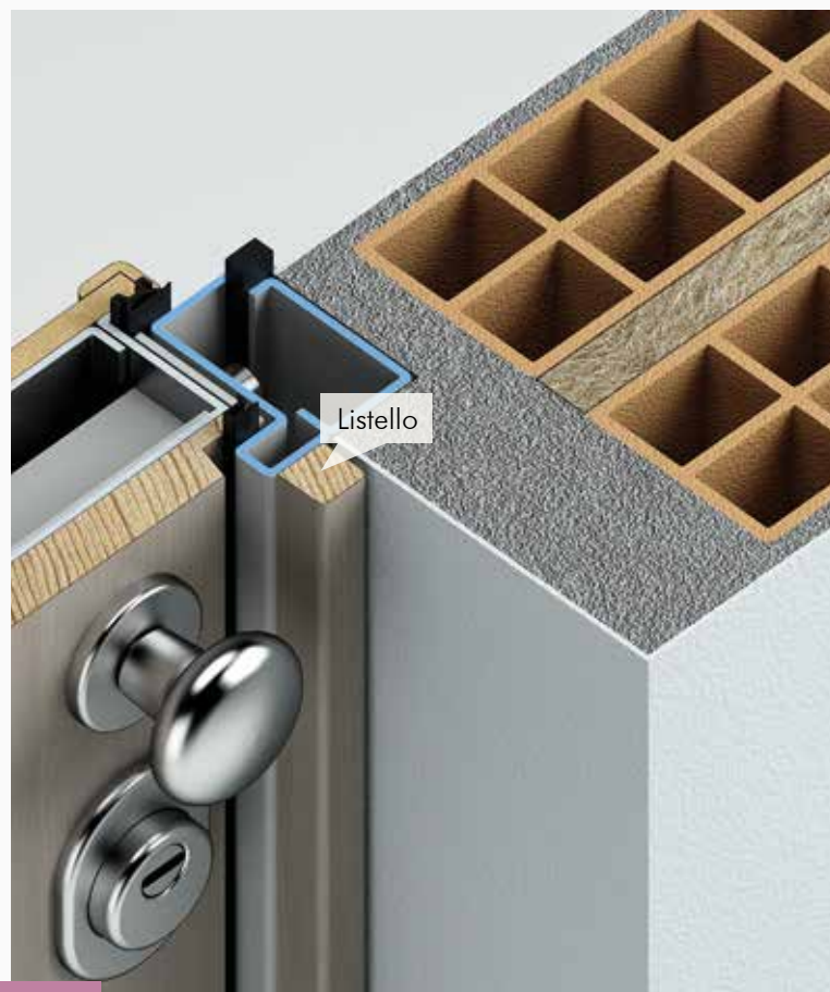
Rifinitura : LISTELLO 2X2 MASSELLO, LACCATO Caratteristica : lo spessore di 2 cm è costante; la larghezza può variare fino a max 15 cm
