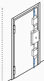
Chiusura testata e chiusura a pavimento
