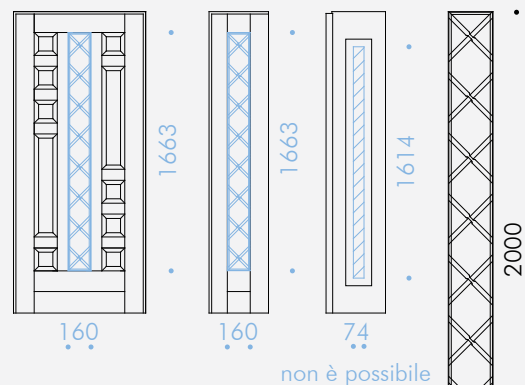
Grata FORATA "D" 25x200
