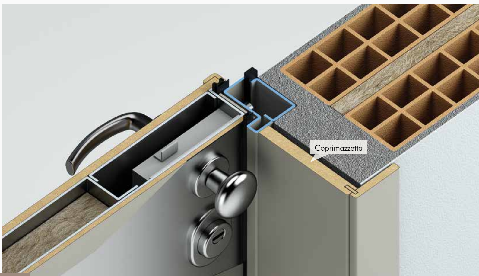
1 Rifinitura : COPRIMAZZETTA CON MOSTRE 7X1 LACCATO Caratteristica : bordo coprimazzetta r3
