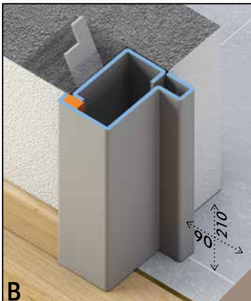
POSA CENTRO MAZZETTA
