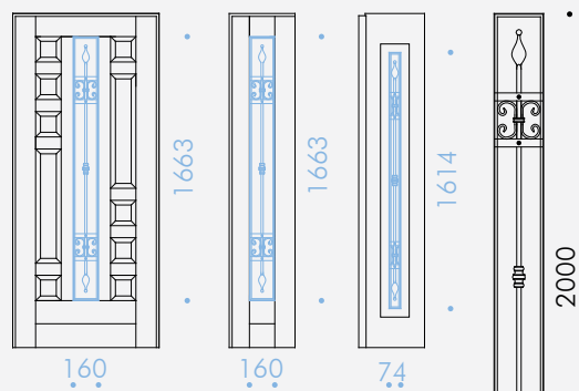
Grata CLASSICA 25x200
