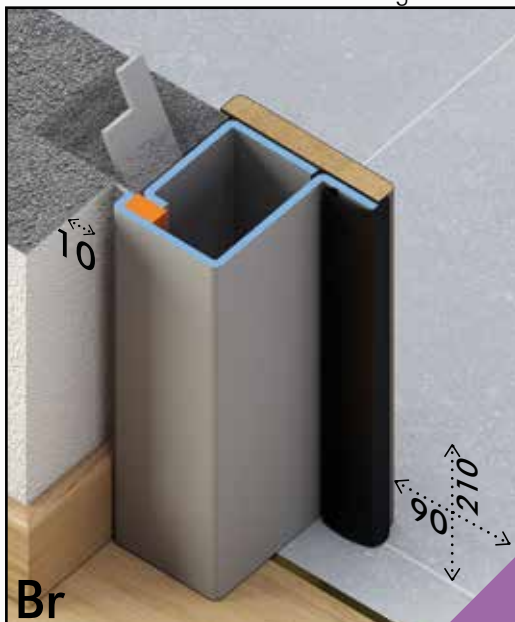
POSA FILO ESTERNO
