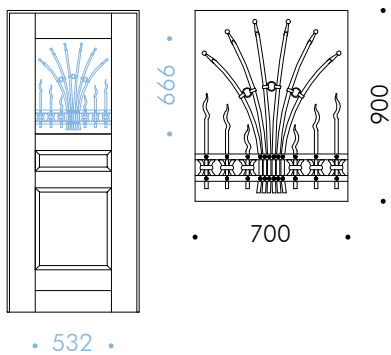
Grata LIBERTY-C 70x90
