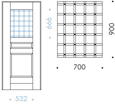
Grata CHIODATA 70x90
